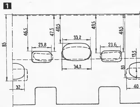
Рис. 1. Развертки цилиндров М-105 (пунктир) и М-106 (сплошная линия).
