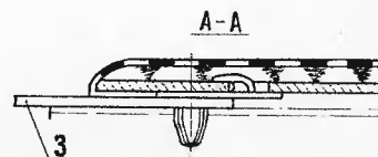
Рис. 1. Контроль за положением дверей и демонтаж обивки: 1 — полоски бумаги; 2 — пластмассовые держатели; 3 — лопатка-съемник.
