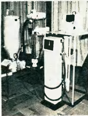
Моечная установка для блоков цилиндров и коленчатых валов автомобильных и тракторных двигателей.
